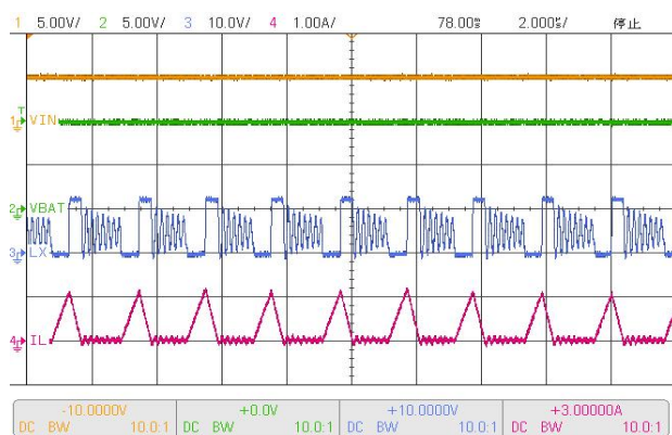
Figure 9.1 各阶段充电开关波形
