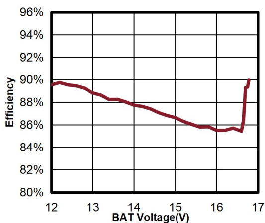
Figure 8.1.a R_{ICHG}=1.3K , 恒流和恒压充电阶段效率
