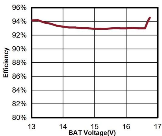
Figure 8.2.a R_{ICHG}=0.5K , 恒流和恒压充电阶段效率
