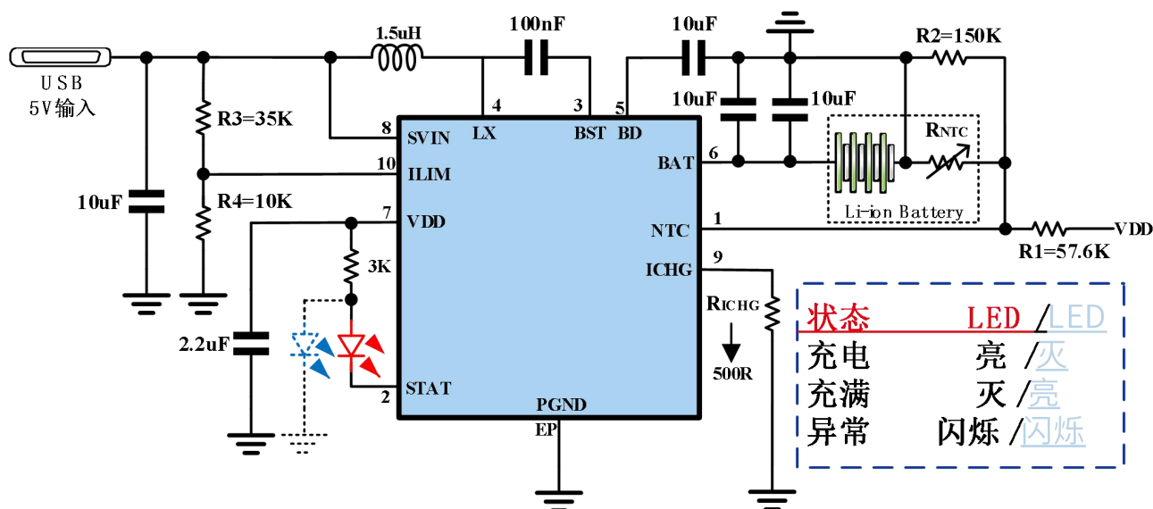
图 2 JZ55184 ESSOP10 版本 USB 5V 适配器充电 (适应最低 4.5V USB 适配器; 电池充电温度为 0℃~60℃)
