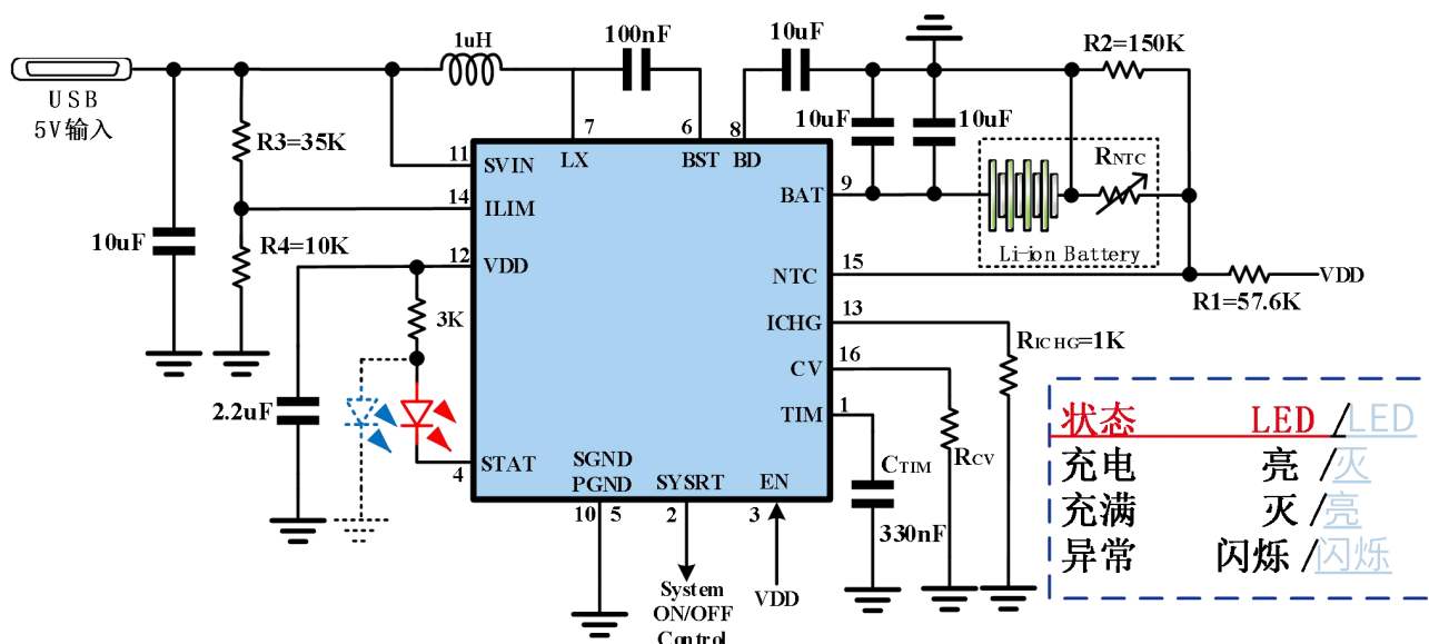
图 1 JZ55184 QFN USB 5V 适配器充电 (适应 4.5V USB; 电池充电温度为 0°C~60°C)
