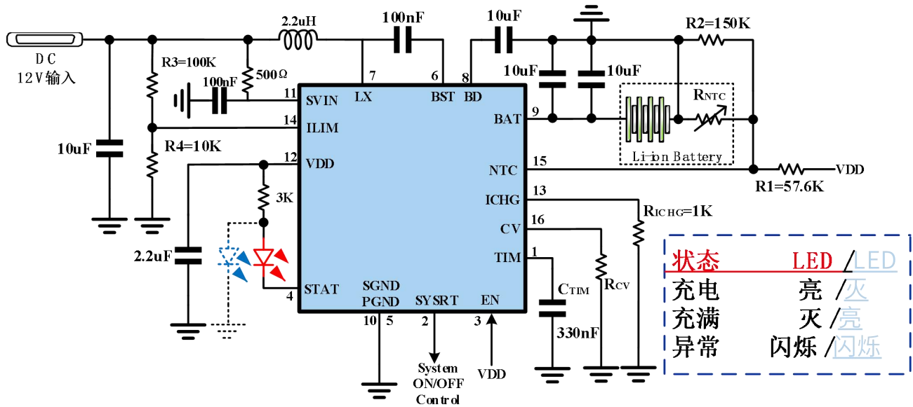
图3 JZ55184 QFN 版本 DC 12V 适配器充电 (适应最低 11V DC 适配器; 电池充电温度为 0°C~60°C)
