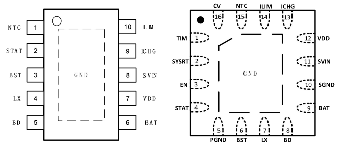
图 4. 引脚排列
